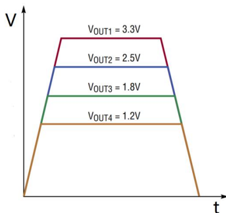
图 6 输出重合跟踪波形
