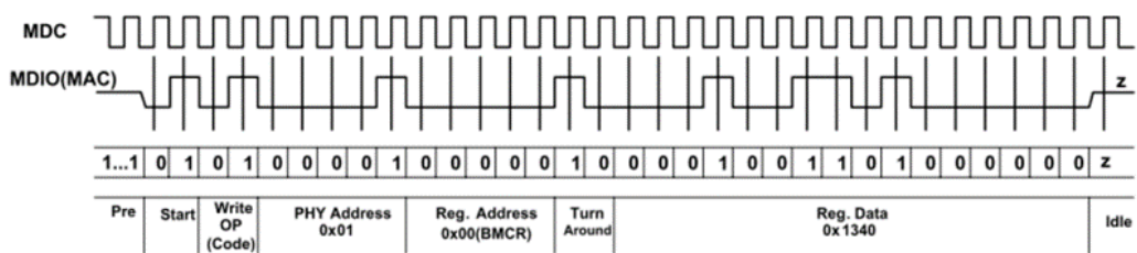
图 26.11 MDC/MDIO 的写数据时序图
