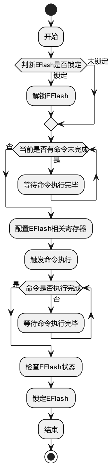
图 5.2 EFLASH 操作流程圖
