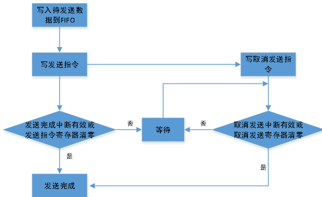
图 21.2 发送数据流程示意图
