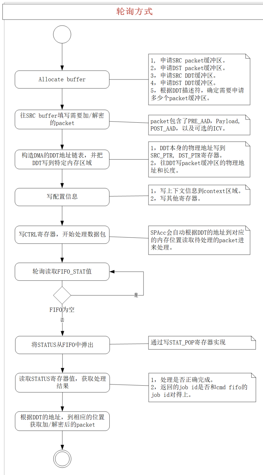
图 31.6 操作流程
