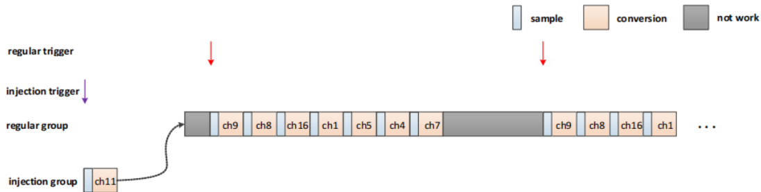
图 29.10 mode3 注入组间隔模式在 ADC 空闲状态下具有注入触发的工作流程图
