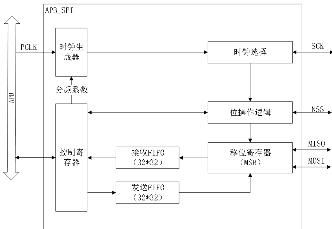
图 23.1 系统框图
