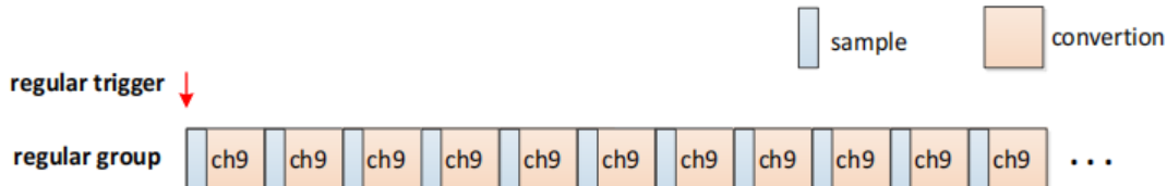
图 29.6 mode2 工作流程图
