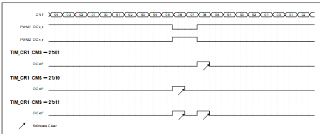
图 24.27 中心对齐模式，中断标志时序图（ARR=07、CCRx=06）
