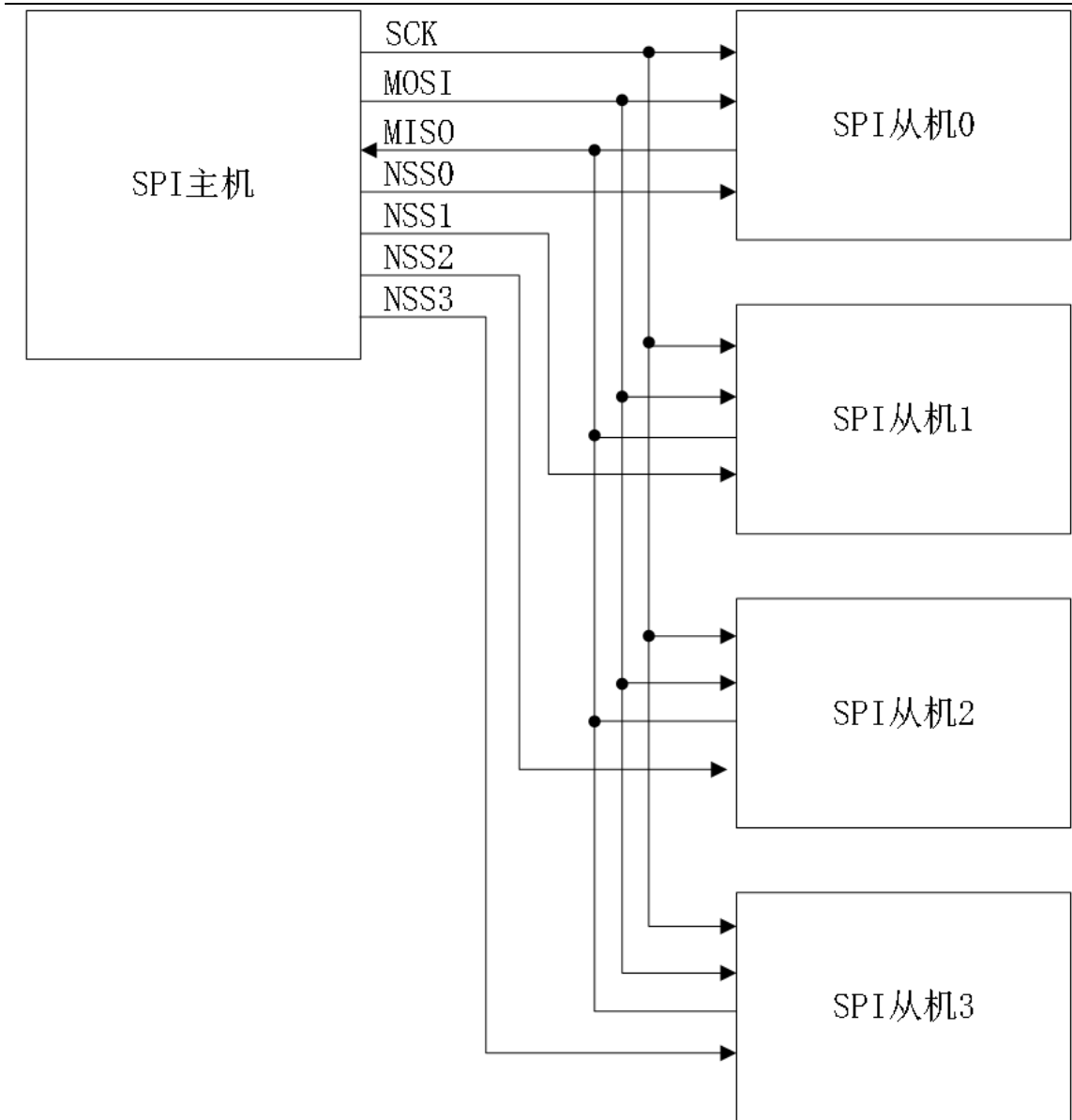
图 23.4 单主多从结构图
