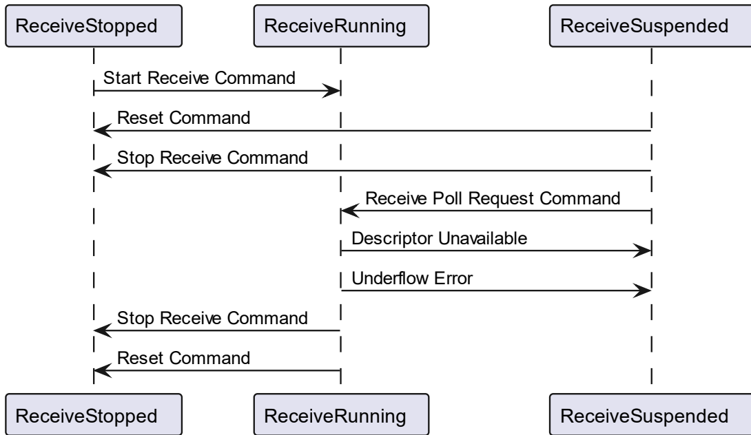
图 26.9 MAC 接收数据状态转换示意图
