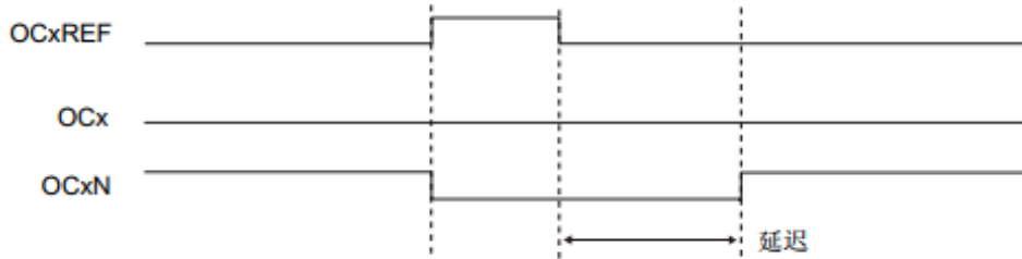
图 24.35 延迟时间大于正脉冲宽度的死区波形图
