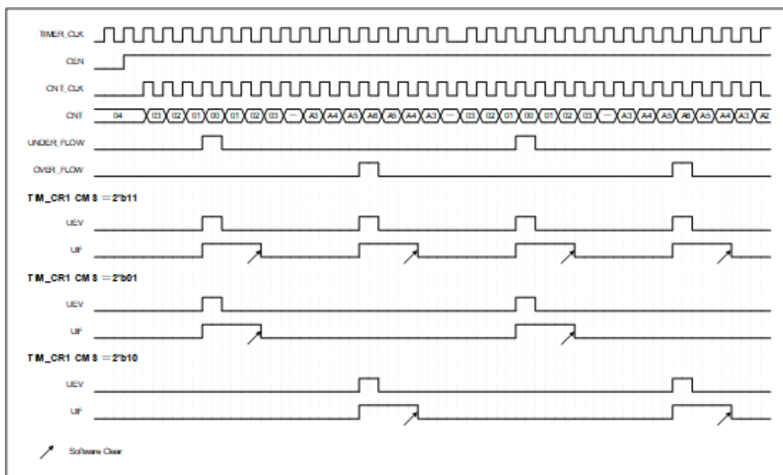
图 25.12 中心对齐模式，计数器时序图
