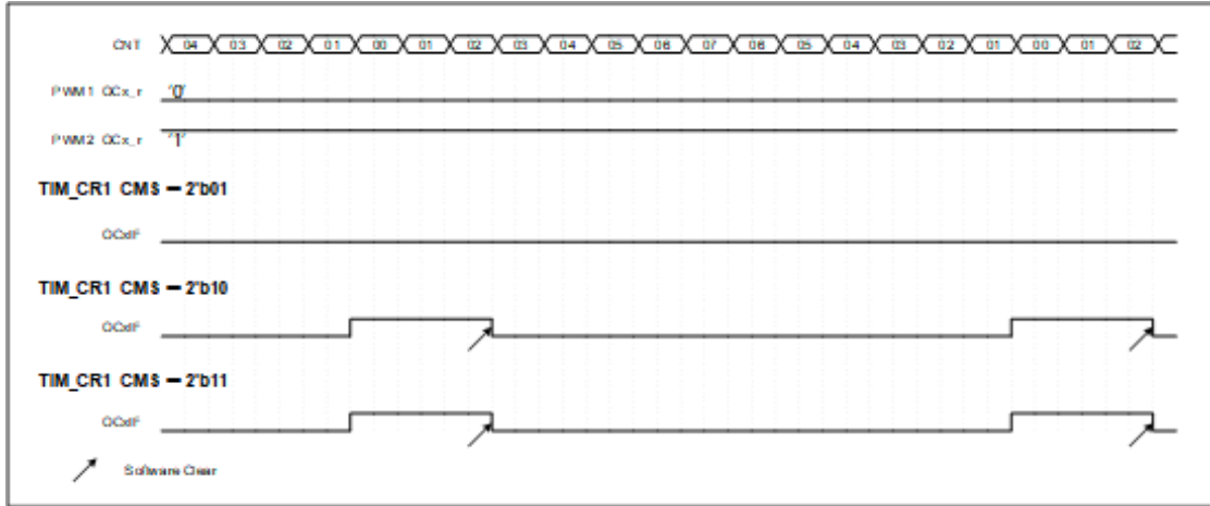
图 24.25 中心对齐模式，中断标志时序图（ARR=07、CCRx=00）
