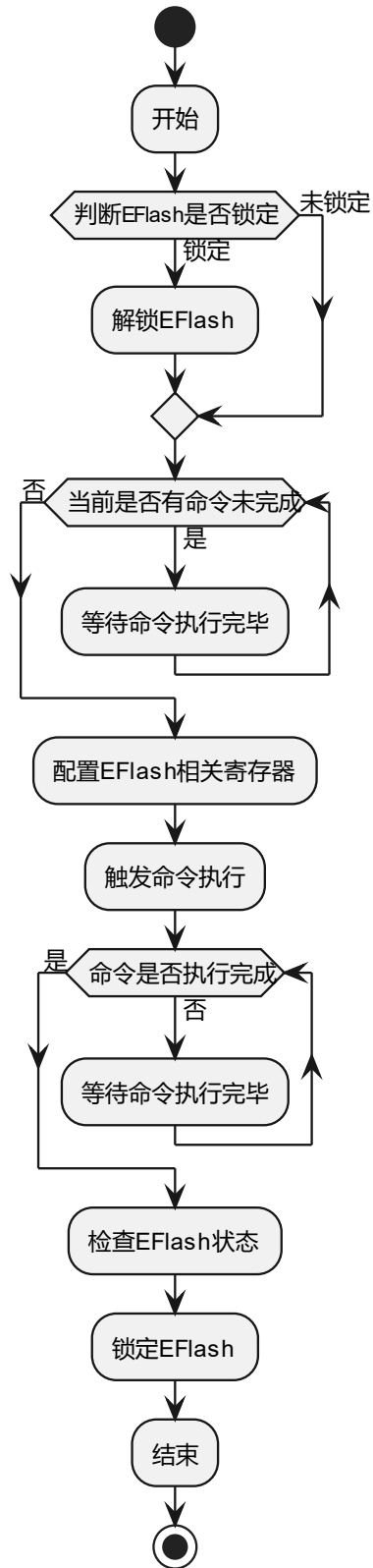
图 5.2 EFLASH 操作流程
