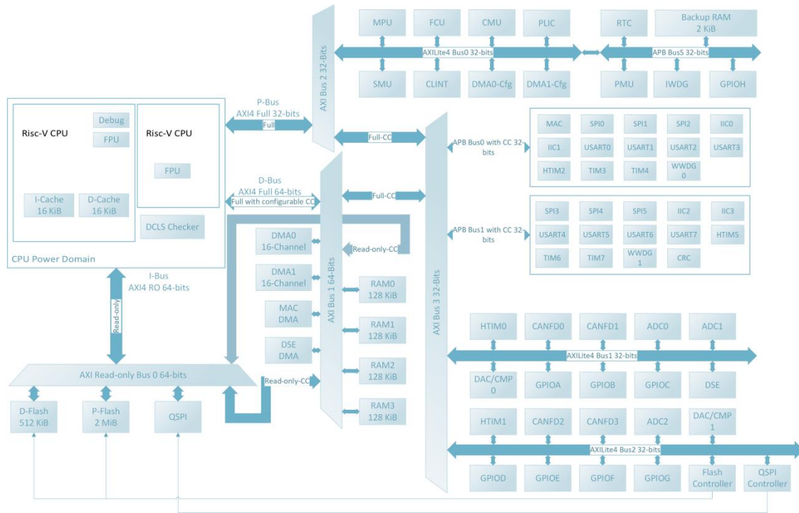
图 1.1 结构框图
