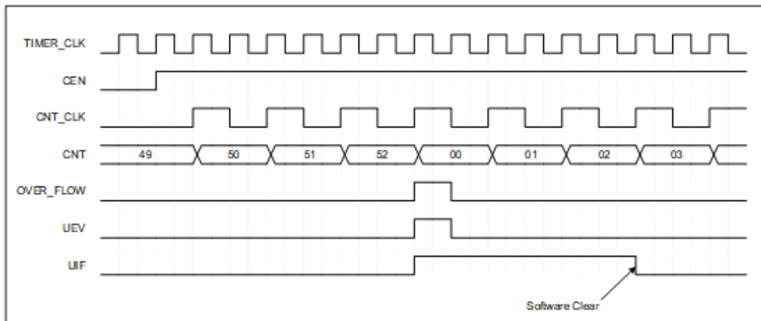
图 24.7 递增计数时序图（2 分频）
