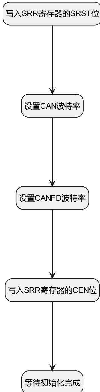
图 21.1 CAN 初始化流程示意图
