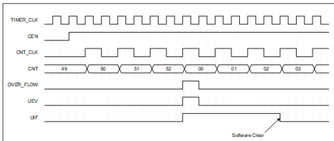
图 25.5 递增计数时序图（2 分频）
