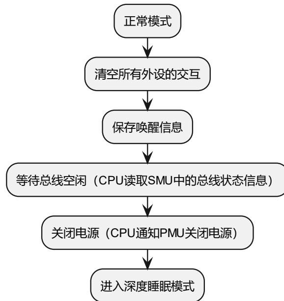
图 8.2 深度睡眠模式的工作流程示意图
