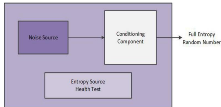
图 31.10 熵源结构图
