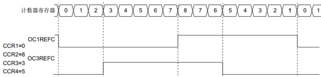
图 24.30 50% 占空比时产生的 2 个相移 PWM 信号
