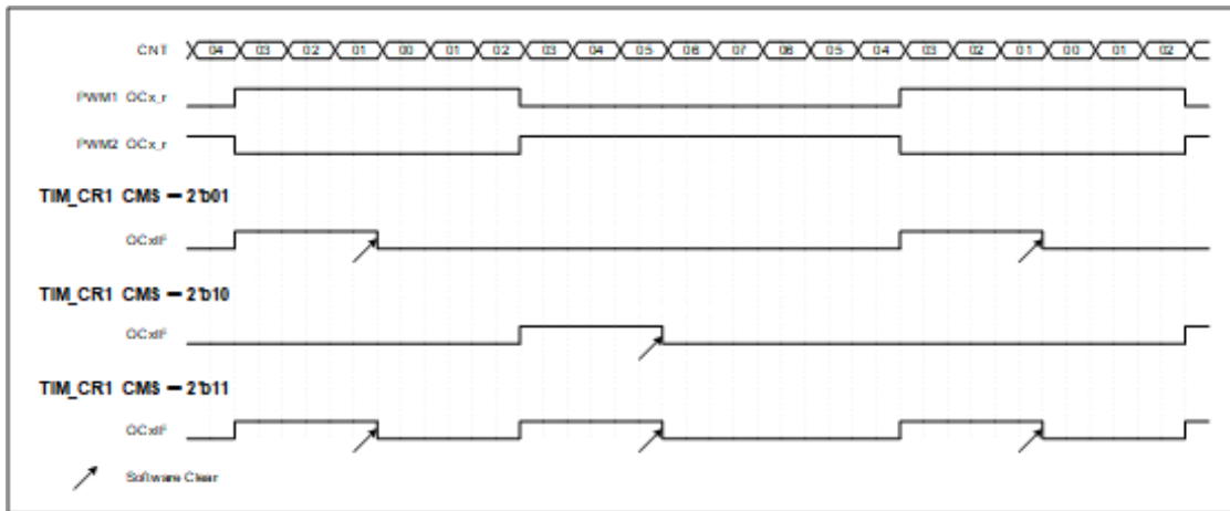
图 24.26 中心对齐模式，中断标志时序图（ARR=07、CCRx=03）
