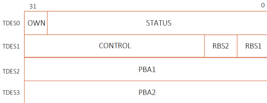
图 26.7 发送描述符的字节组成示意图
