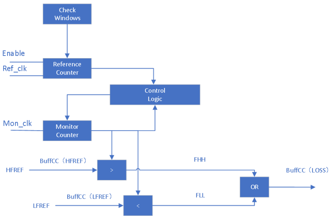
图 18.1 结构框图
