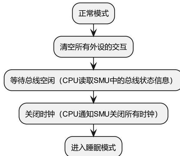
图 8.1 睡眠模式的工作流程示意图
