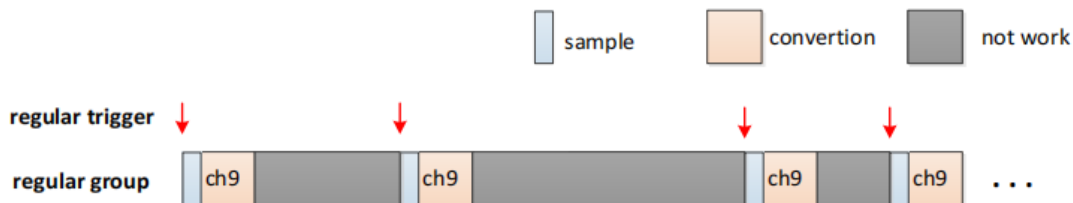
图 29.5 mode1 工作流程图
