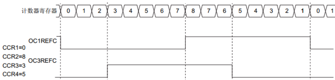
图 25.27 50% 占空比时产生的 2 个相移 PWM 信号
