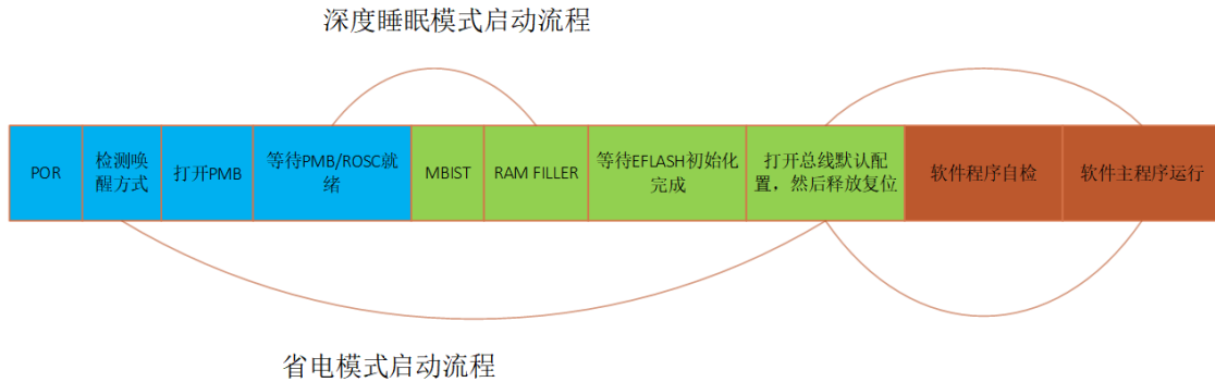
图 4.4 上电流程
