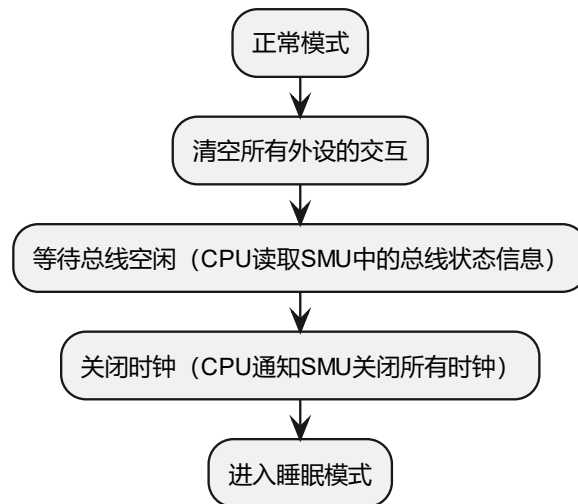
图 8.1 睡眠模式的工作流程示意图
