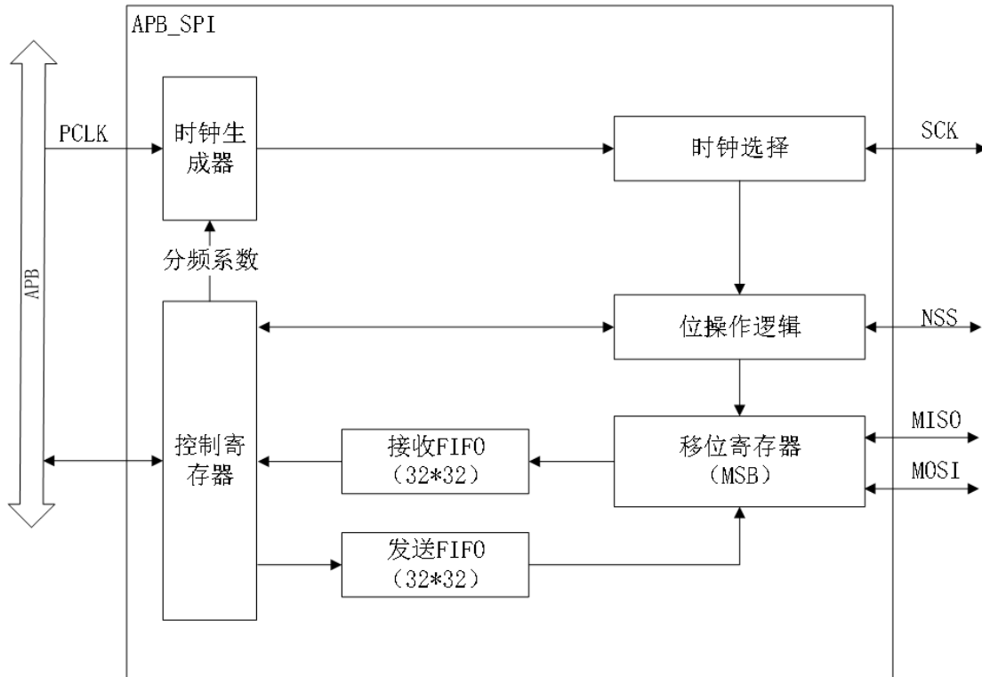
图 23.1 系统框图
