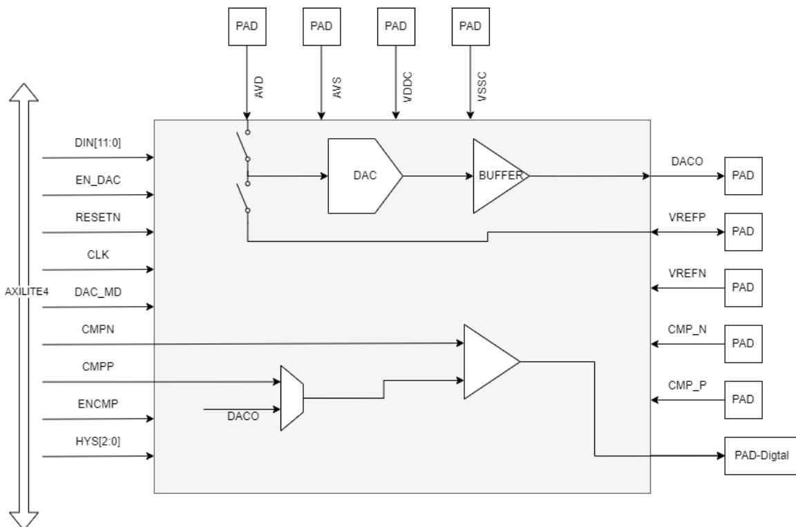
图 30.1 DAC 结构框图
