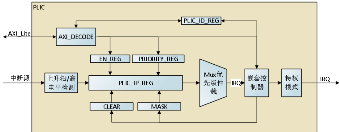
图 11.1 PLIC 架构示意图
