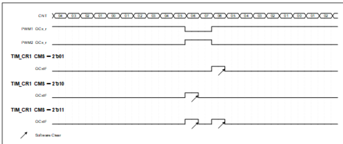
图 25.24 中心对齐模式，中断标志时序图（ARR=07、CCRx=06）
