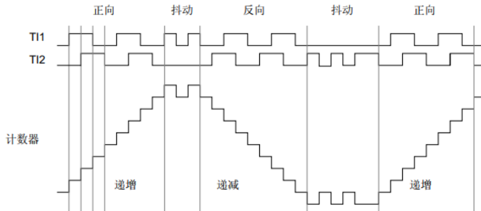
图 24.16 编码器模式下计数器工作示意图
