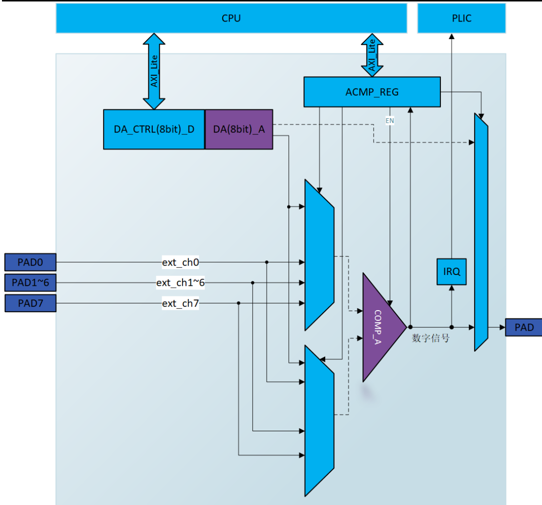
蓝色部分为数字电路，紫色部分为模拟电路
