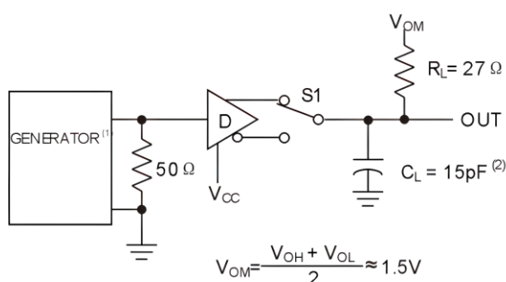
图 14 驱动器传播时间
