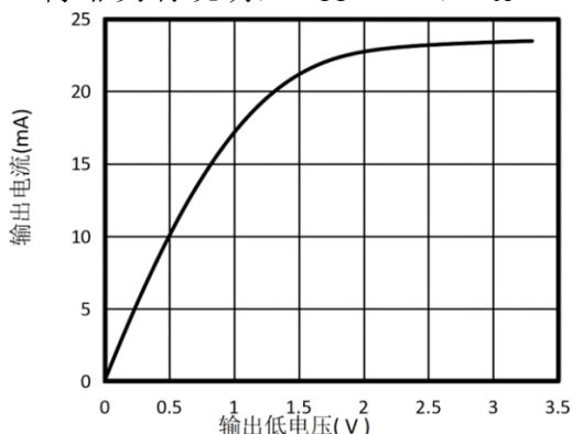
图 1. 输出电流与接收器输出低电压
