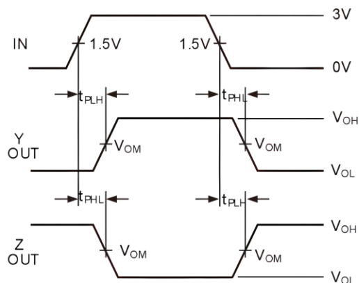
图 14 驱动器传播时间
