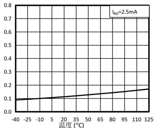
图 4. 接收器输出低电压与温度
