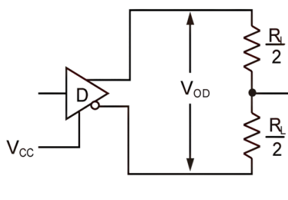
图 10 驱动器 V_{OD} 和 V_{OC}
