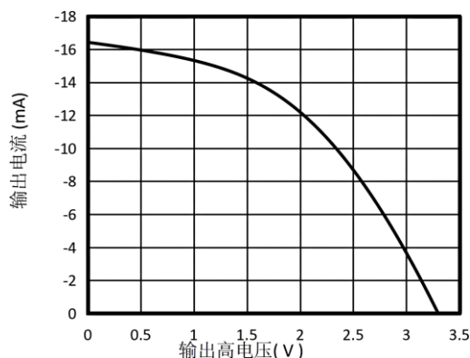
图 2. 输出电流与接收器输出高电压
