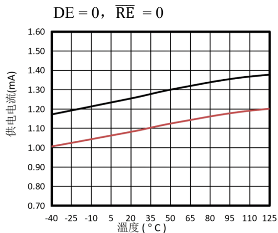
图 9. 电源电流与温度
